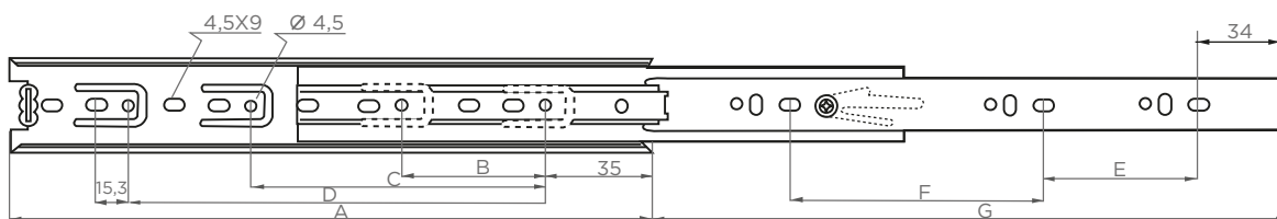
Diagrama de producto e instalación
